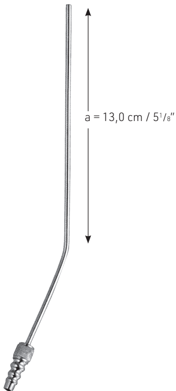
YASARGIL 017-470-015 Ø 1,5 mm 017-470-020 Ø 2,0 mm 017-470-025 Ø 2,5 mm 017-470-035 Ø 3,5 mm
